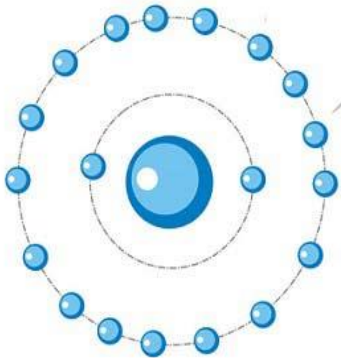
АНТИОКСИДАНТ
