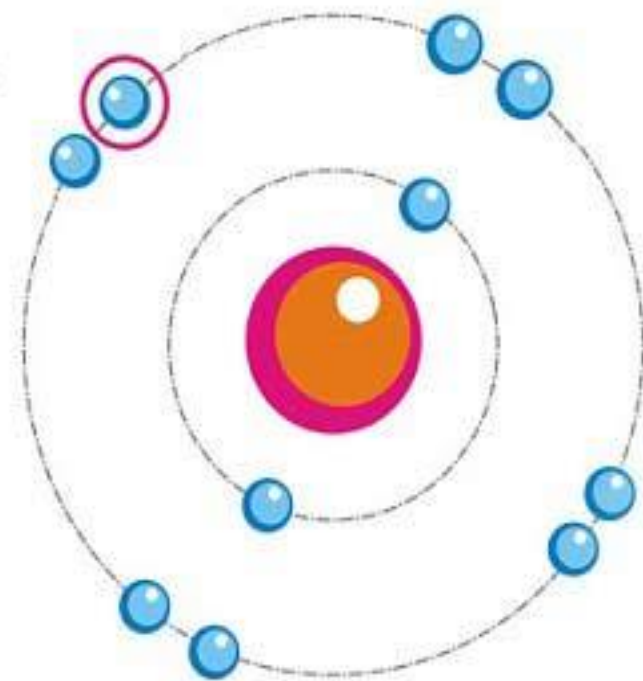
СВОБОДНЫЙ РАДИКАЛ
